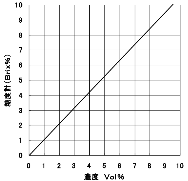
リライアソルE-Bの濃度換算グラフ
